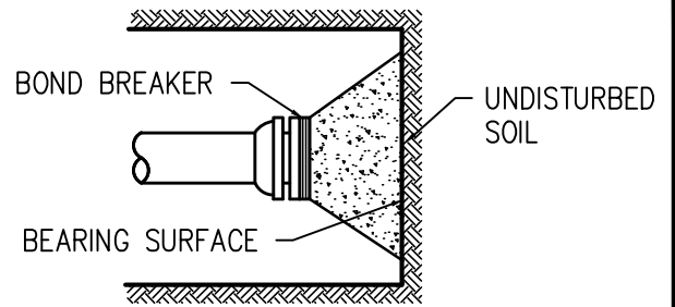
DEAD END
