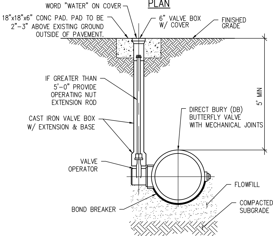
ELEVATION
